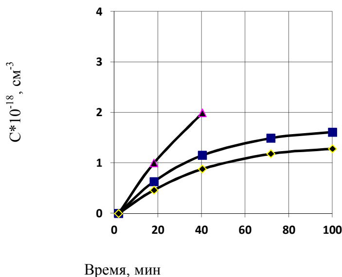
Рис.2. Зависимость концентрации накопления молекулярных продуктов ( 1720\text{ см}^{-1} ) от времени при механической нагрузке \sigma = 15\text{ кг/мм}^2 , T = 20^\circ\text{C} , □- пленки толщиной 60\text{ мкм} , соответственно не стабилизировано, △ - то же самое с диафеном НН и ◇ - трисалкофен БМБ.
