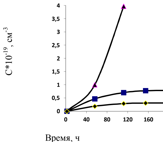
Рис.1. Зависимость концентрации накопления молекулярных продуктов ( 1720\text{ см}^{-1} ) от времени при T=120^\circ\text{C} , □ - пленки толщиной 60\text{ мкм} , соответственно не стабилизировано, △ - то же самое с диафеном НН и ◇ - трисалкофен БМБ.
